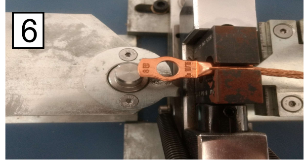
Lug Crimping
